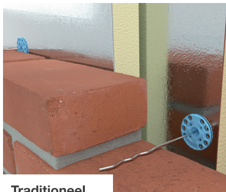
Traditioneel metselwerk
