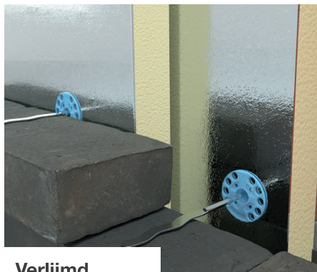
Verlijmd metselwerk
